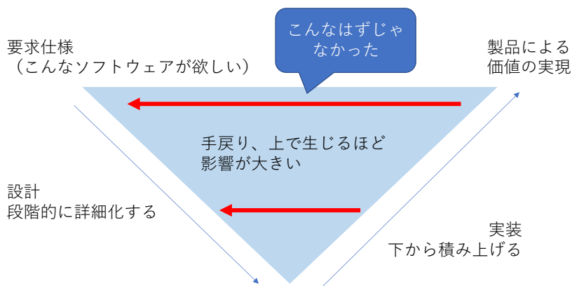
図 49 ソフトウェア開発の V モデル
